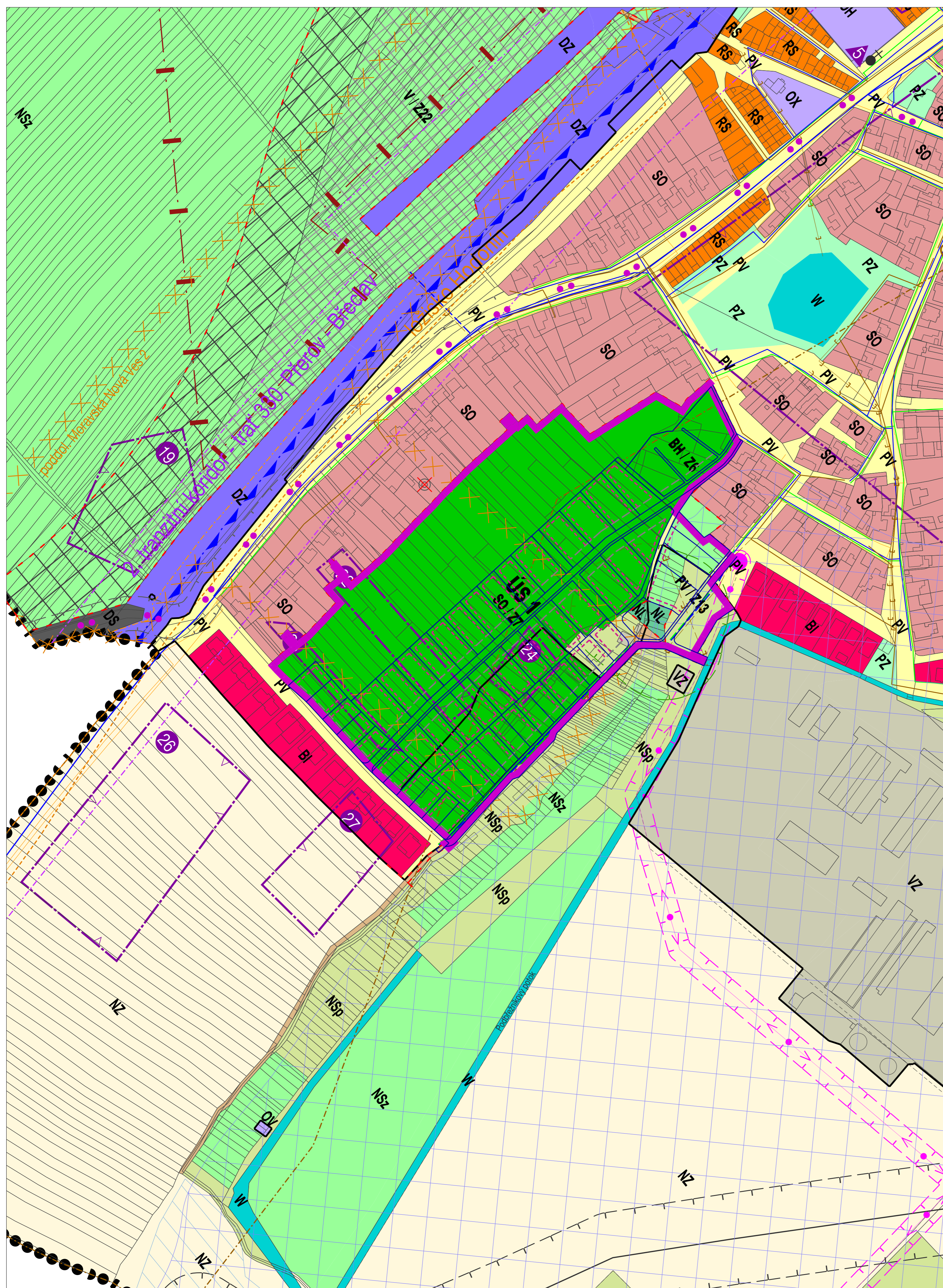
DETAIL KOORDINAČNÍHO VÝKRESU ÚZEMNÍHO PLÁNU
